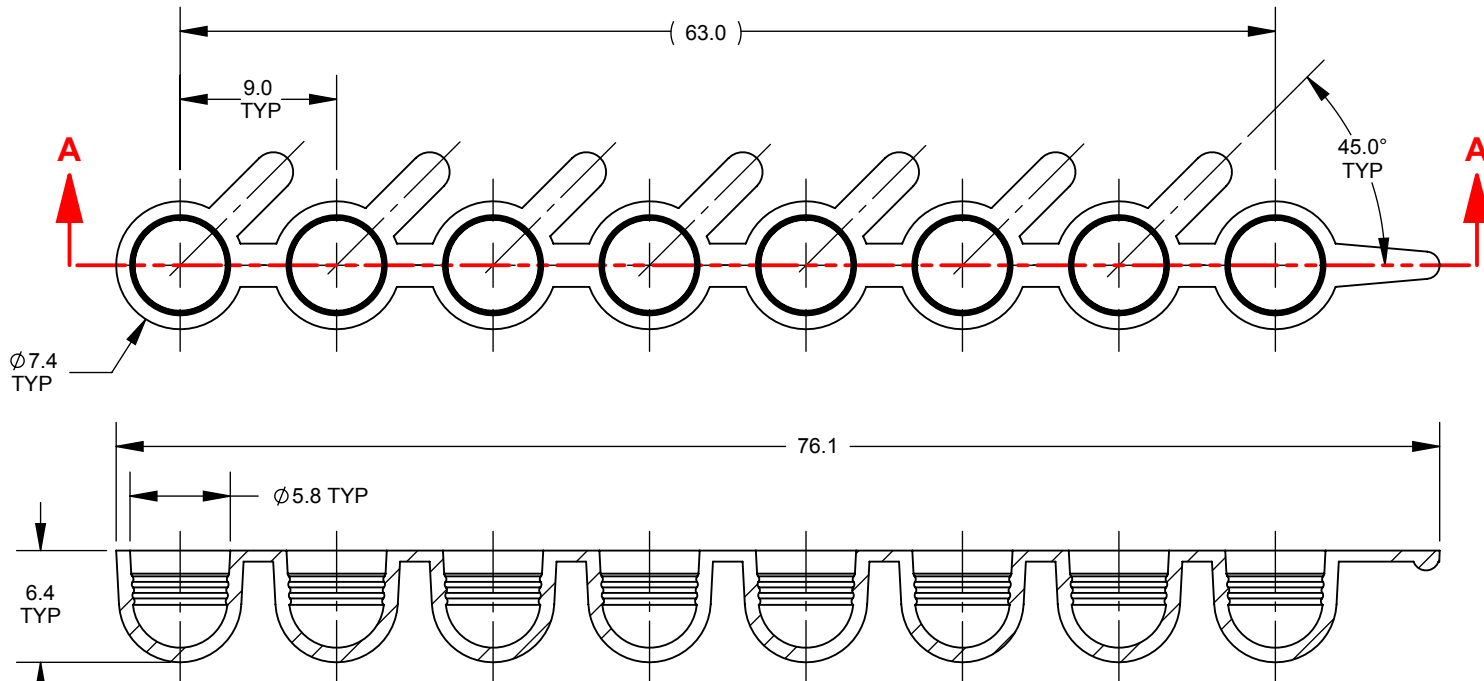
SECTION A-A SCALE: 2.3 : 1
