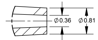
DETAIL B SCALE: 15 : 1
