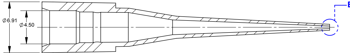
SECTION A-A SCALE: 4 : 1
