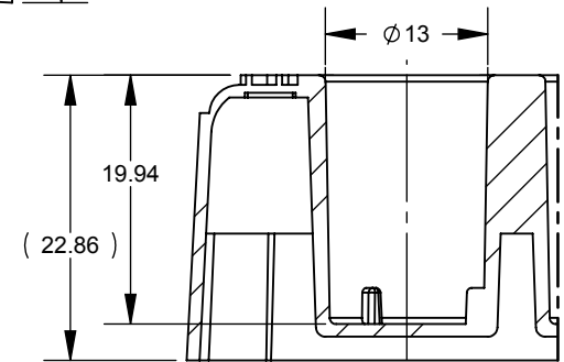
DETAIL B SCALE: 1.5 : 1 TYP
