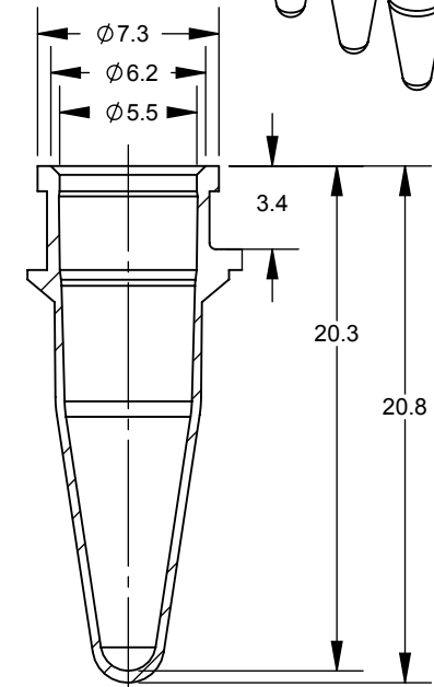
DETAIL B SCALE: 3 : 1 TYP
