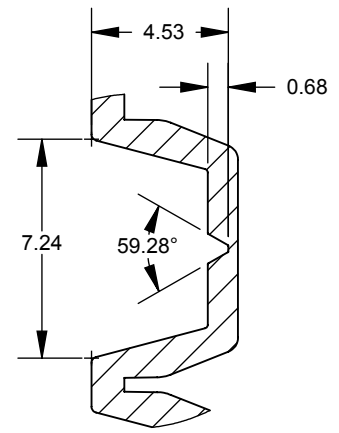
DETAIL D SCALE: 4 : 1 TYP
