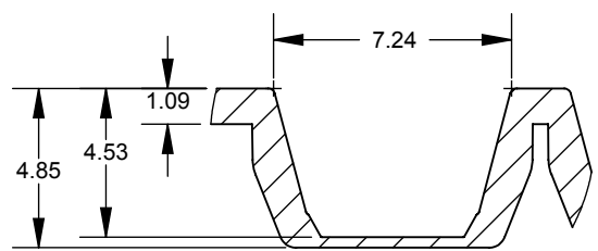
DETAIL C SCALE: 4 : 1 TYP
