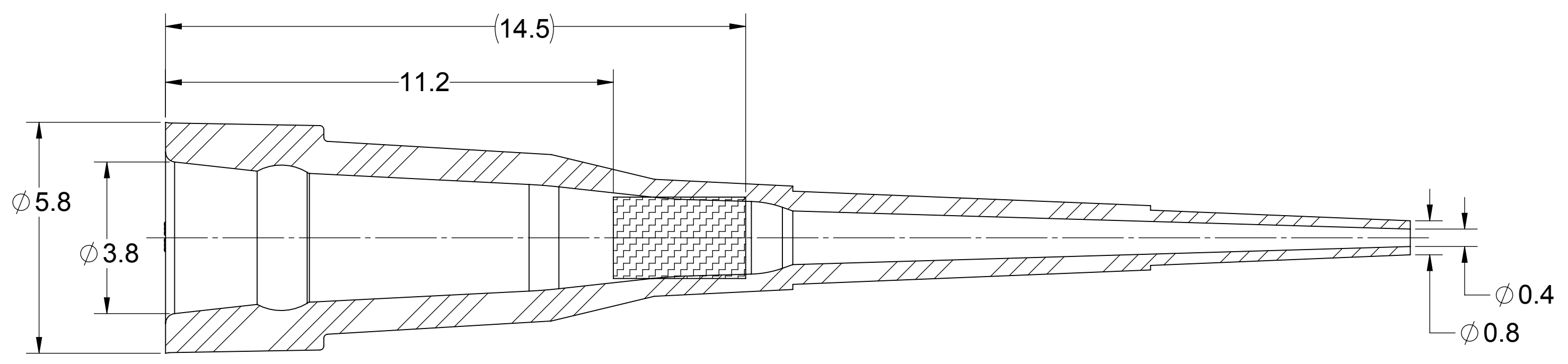
SECTION A-A
