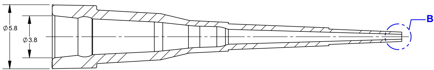
SECTION A-A
