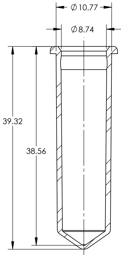
SECTION A-A SCALE: 2.2 : 1
