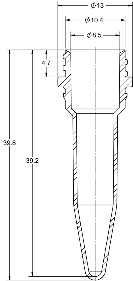
SECTION A-A SCALE: 5 : 1
