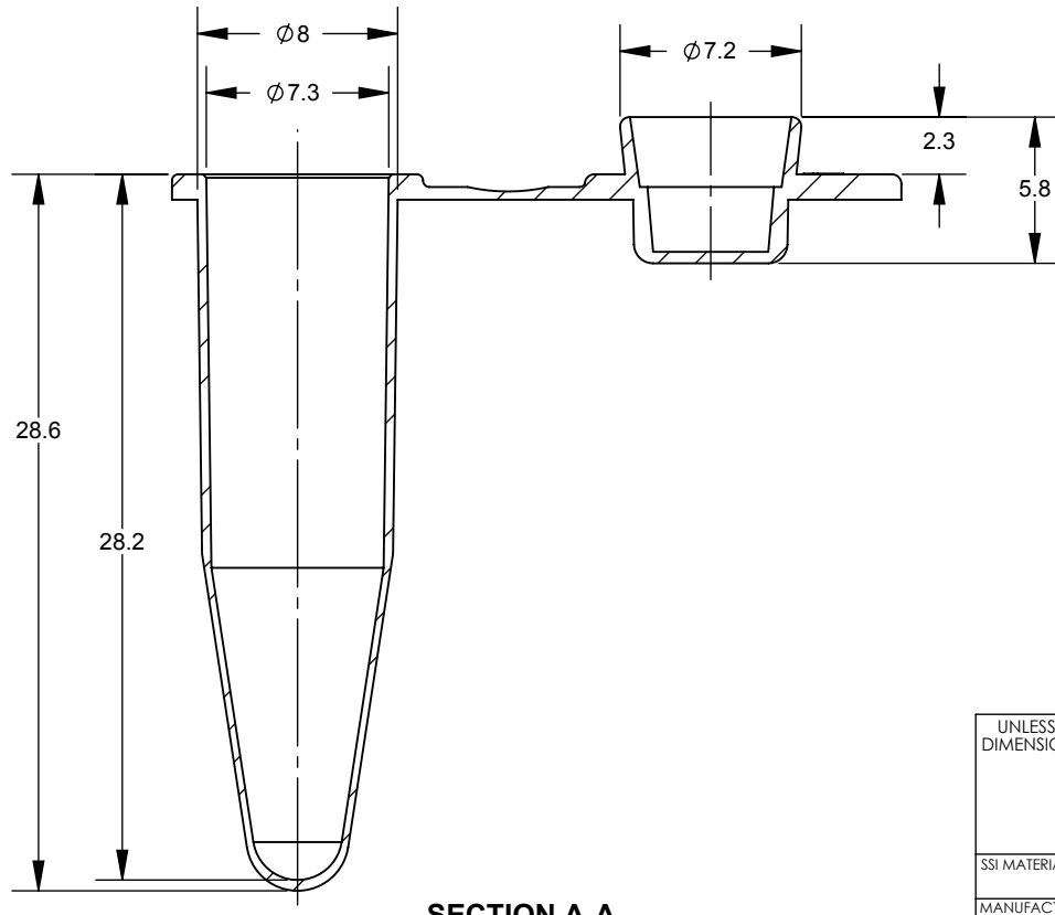
SECTION A-A SCALE: 3 : 1
