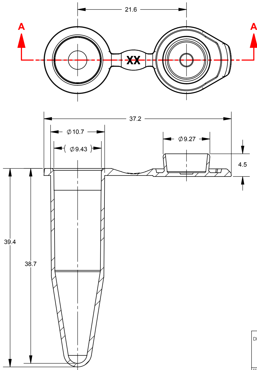
SECTION A-A SCALE: 2.3 : 1
