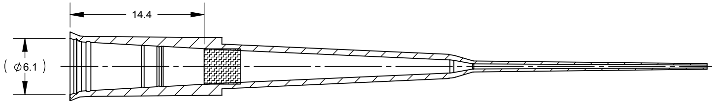
SECTION A-A SCALE: 2.5 : 1
