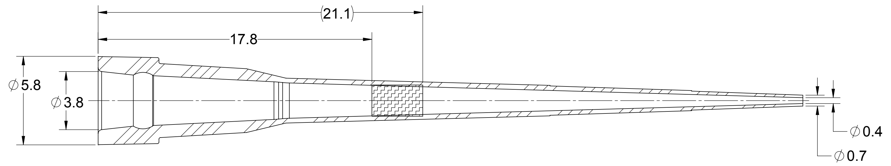
SECTION A-A
