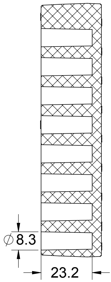
SECTION A-A
