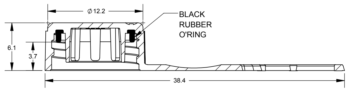
SECTION A-A SCALE: 3.5 : 1
