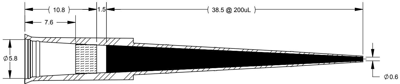
SECTION A-A SCALE: 3 : 1
