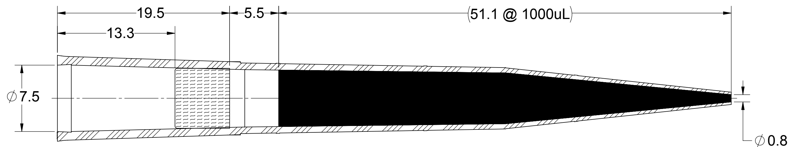
SECTION A-A SCALE: 4 : 1
